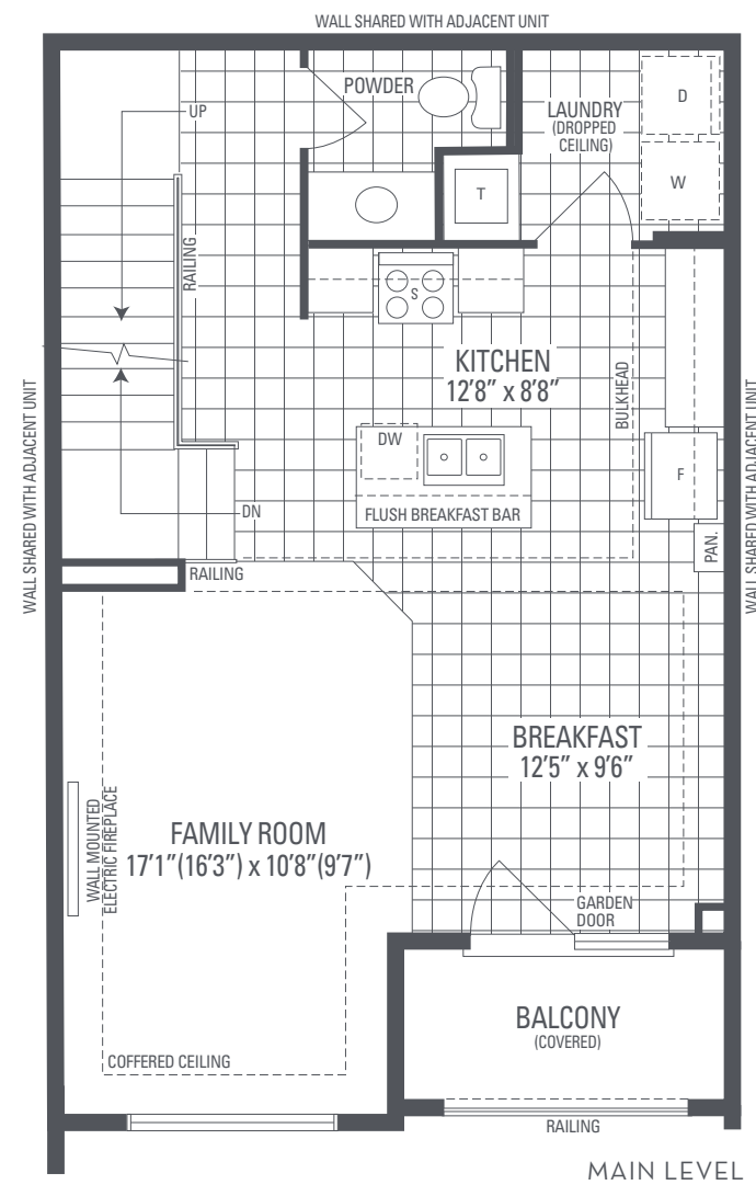
ELEV. 1 & 2
