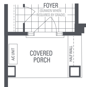
ELEV. 2
